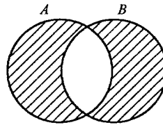
C = A \Delta B Рис. 4
